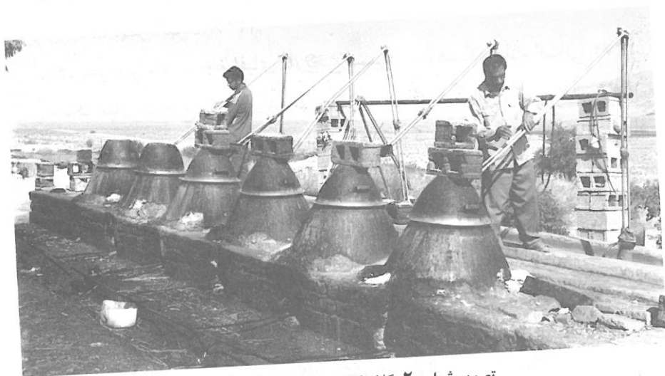
تصویر شماره ۲ - گلاب‌گیری نیمه صنعتی - قمصر
